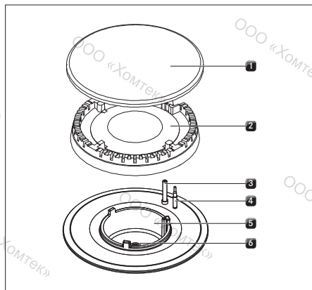
рис. 8.5 Монтаж газовой горелки
