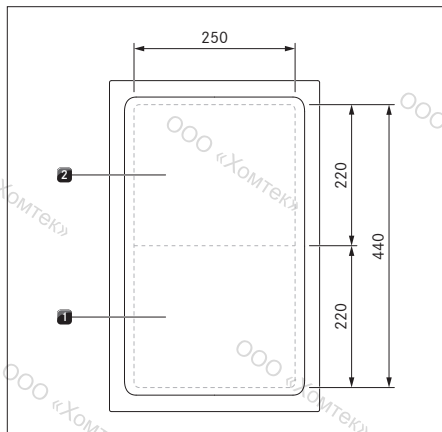
рис. 4.19 Размер конфорок
