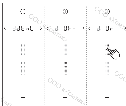
рис. 7.3 Пункт меню D: Активация режима демонстрации
