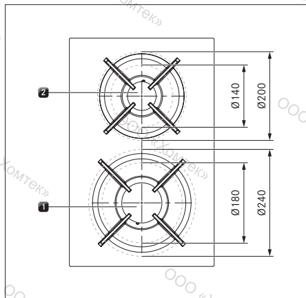
рис. 4.17 Размер конфорок
