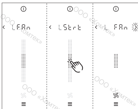
рис. 7.8 Индикация запуска конфигурации вентилятора
