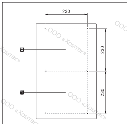
рис. 4.7 Размер конфорок
