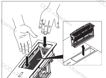
рис. 8.2 Снятие блока жирового фильтра
