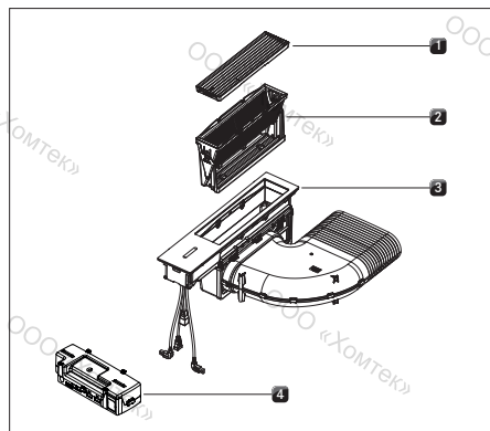
рис. 4.5 BORA Classic вытяжка СКА2/ BORA Classic вытяжка All Black СКА2AB
