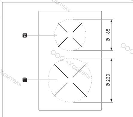
рис. 4.9 Размер конфорок
