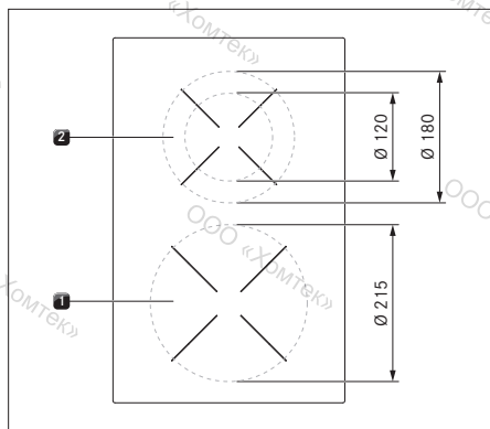
рис. 4.13 Размер конфорок
