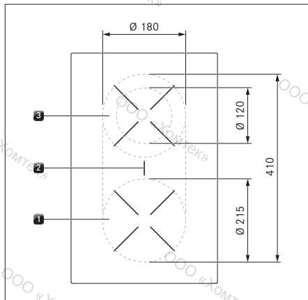
рис. 4.15 Размер конфорок
