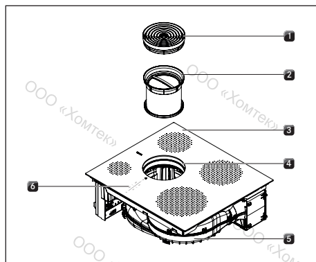
рис. 5.1 Варочная панель
