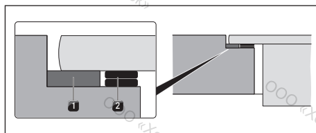
рис. 10.28 Пластины для выравнивания по высоте
