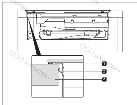
рис. 10.13 Крепление варочной панели по центру
