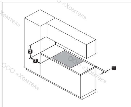
рис. 10.3 обязательные безопасные расстояния
