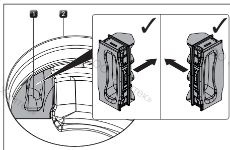
рис. 10.34 Установка откидной крышки фильтра
