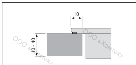
рис. 10.8 Размеры основания для навесного монтажа
