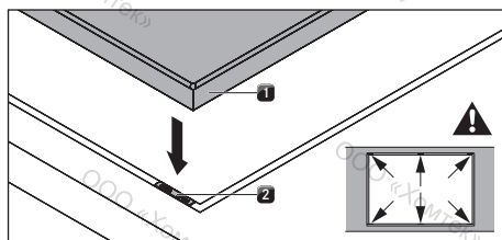
рис. 10.14 Установка пластин для выравнивания по высоте
