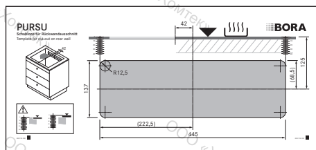
рис. 10.22 Шаблон для выреза в задней стенке
