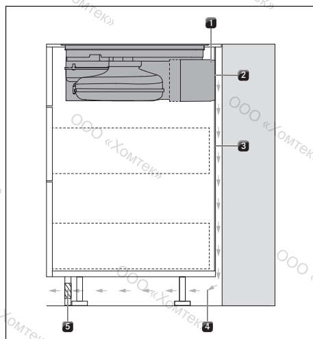
рис. 10.18 Вариант монтажа для сплошной задней стенки
