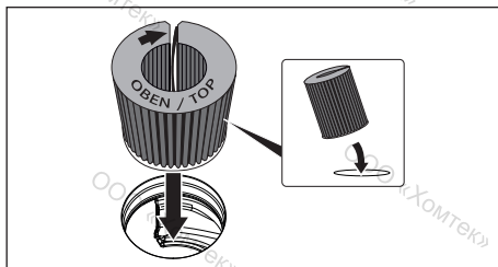
рис. 10.32 Вставьте фильтр с активированным углем в вытяжное отверстие.
