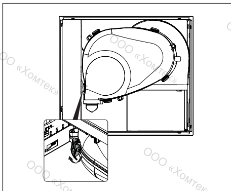
рис. 10.35 Замки камеры всасывания
