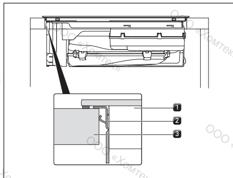
рис. 10.26 Крепление варочной панели
